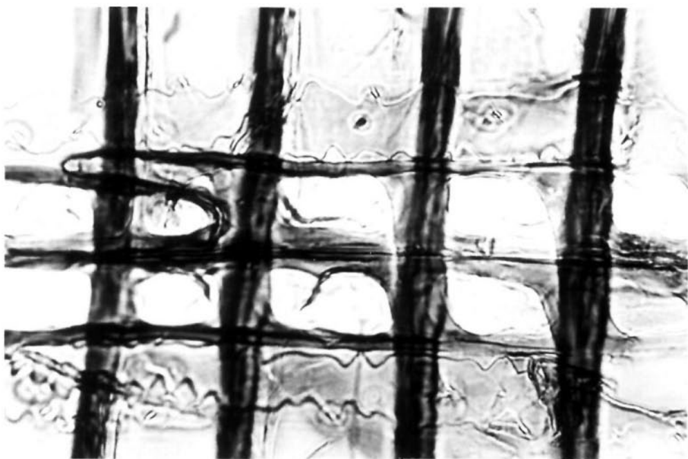
Fig. 3.—Vista en sección radial de los campos de cruce y punteaduras tipo pinoide I. Se aprecian las traqueidas radiales de dientes obtusos. ( \times 500 .)
